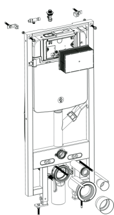
Modul WG-MS100
