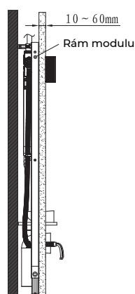
Profil modulu
